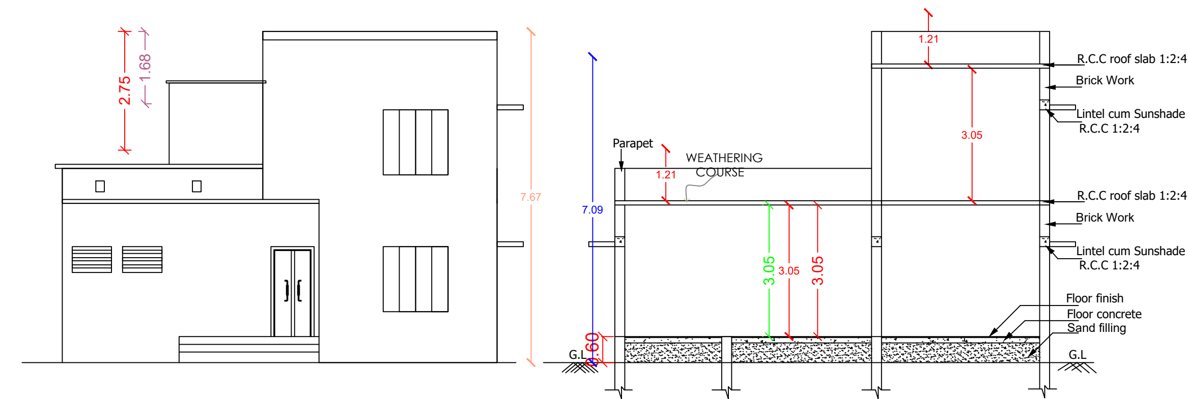
ELEVATION
