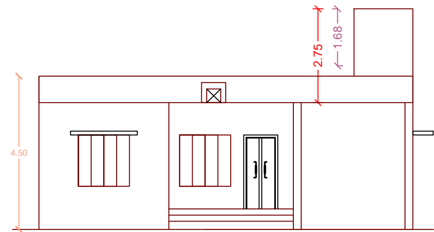
ELEVATION
