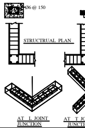
HORIZONTAL SEISMIC
