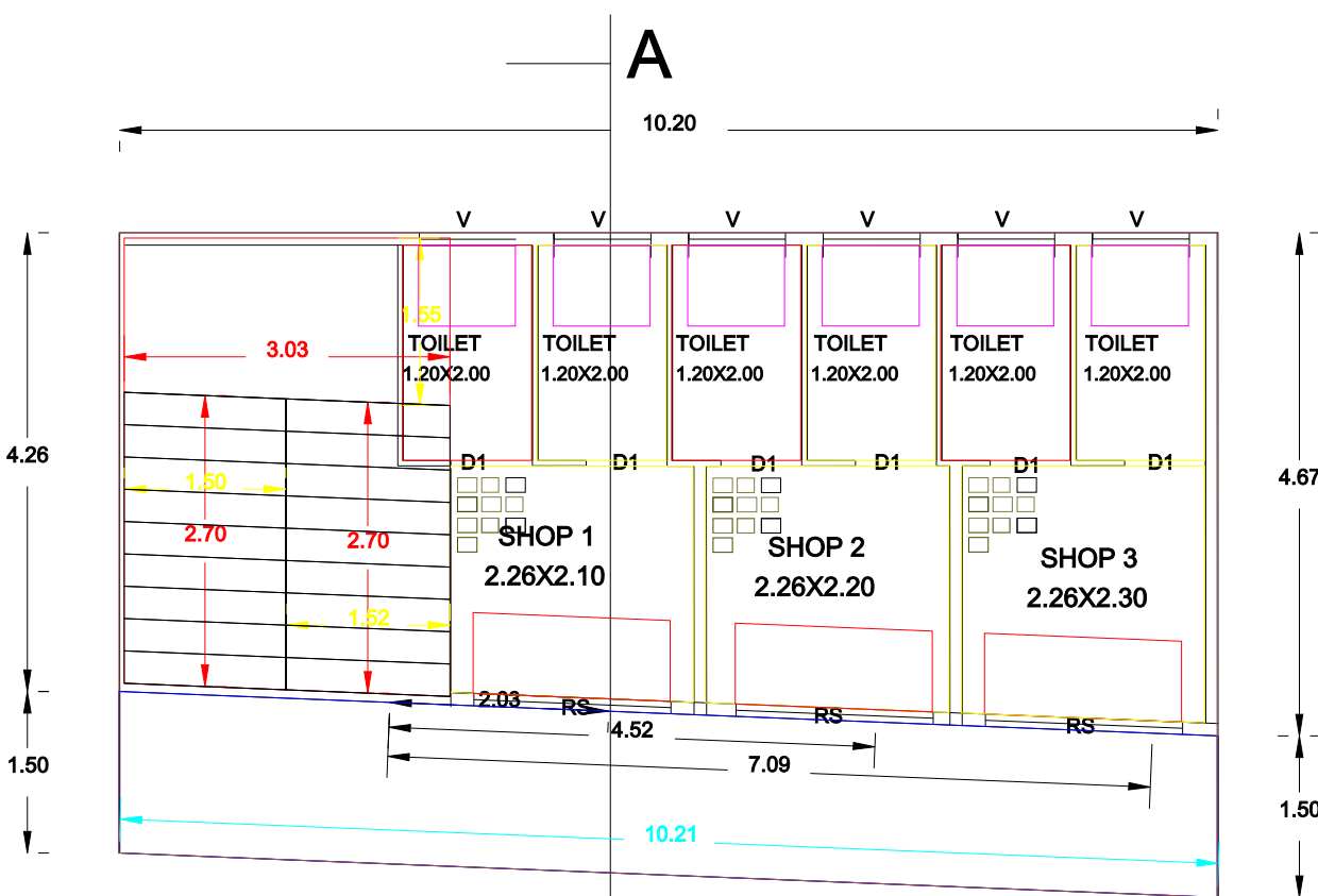
PRO F.FLOOR PLAN
