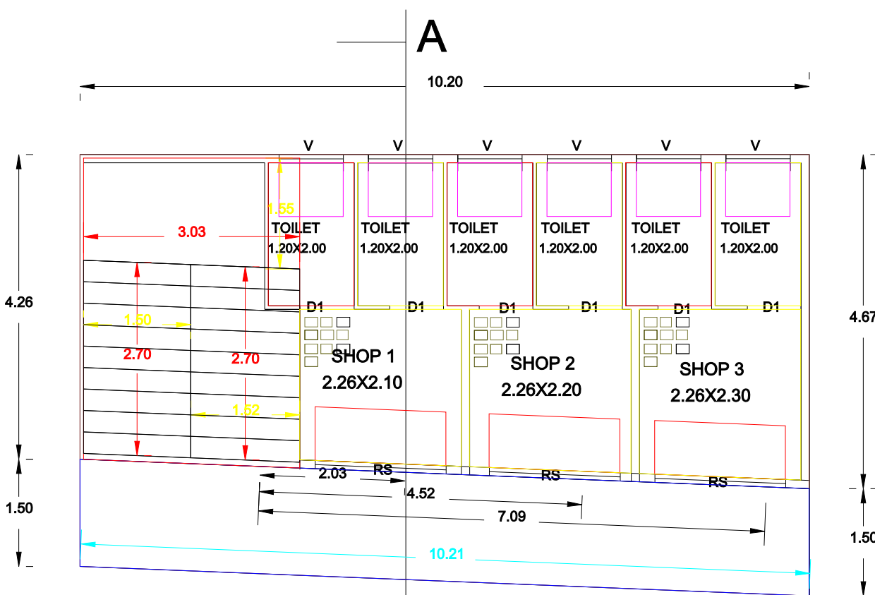
PRO G.FLOOR PLAN
