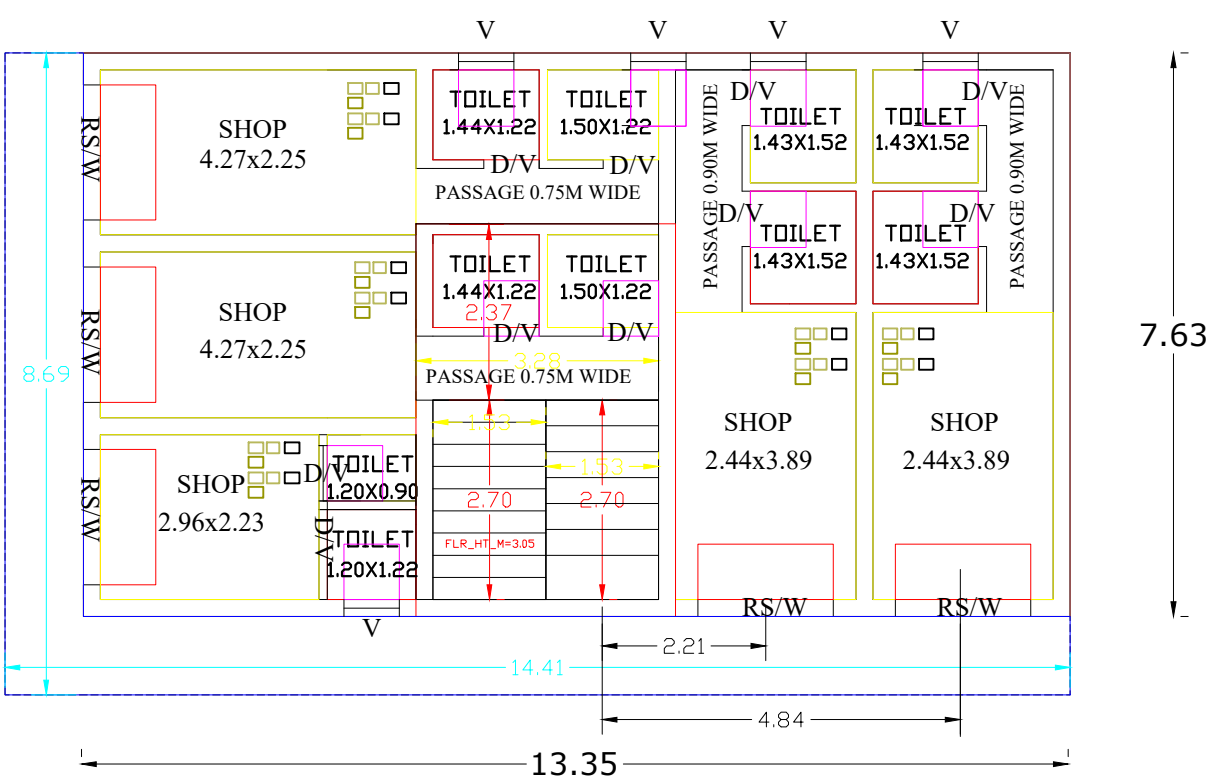
PRO G.FLOOR PLAN
