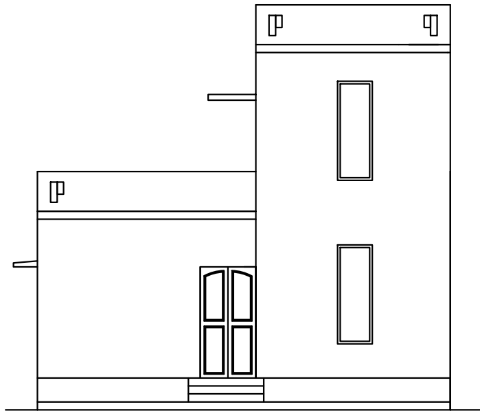
ELEVATION
