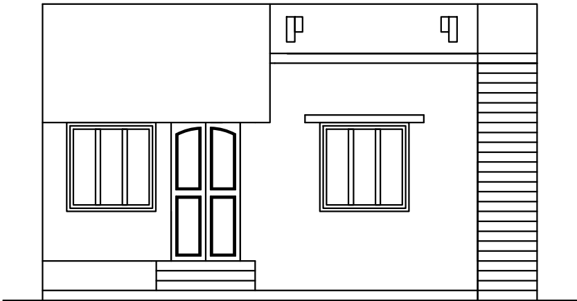
ELEVATION
