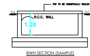
RWH_CAPACITY_L=4800LTRS
