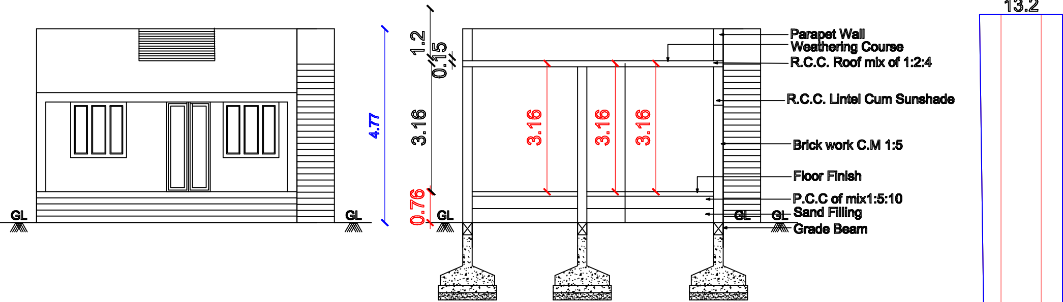
ELEVATION
