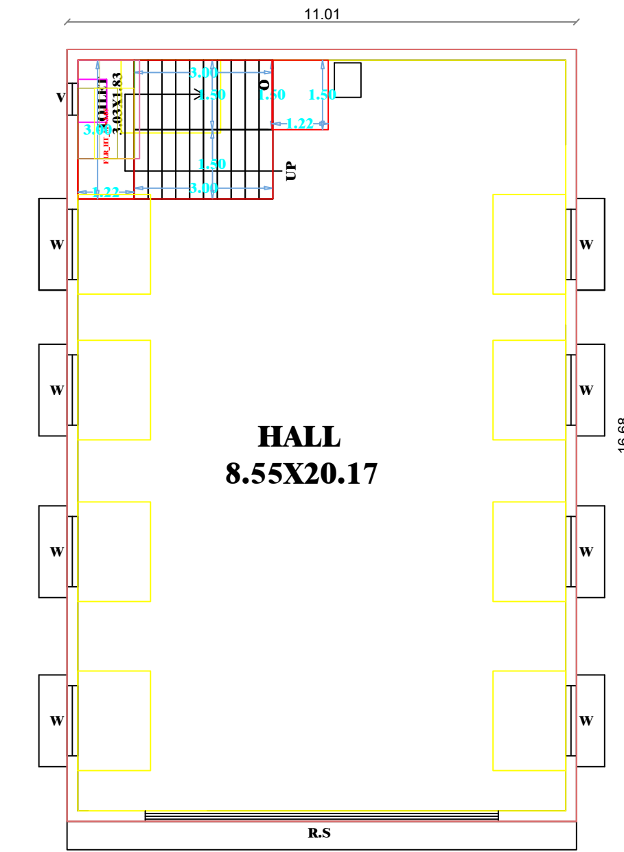
DOOR PLAN
