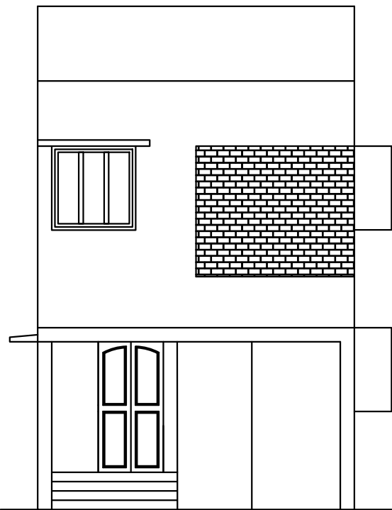
ELEVATION
