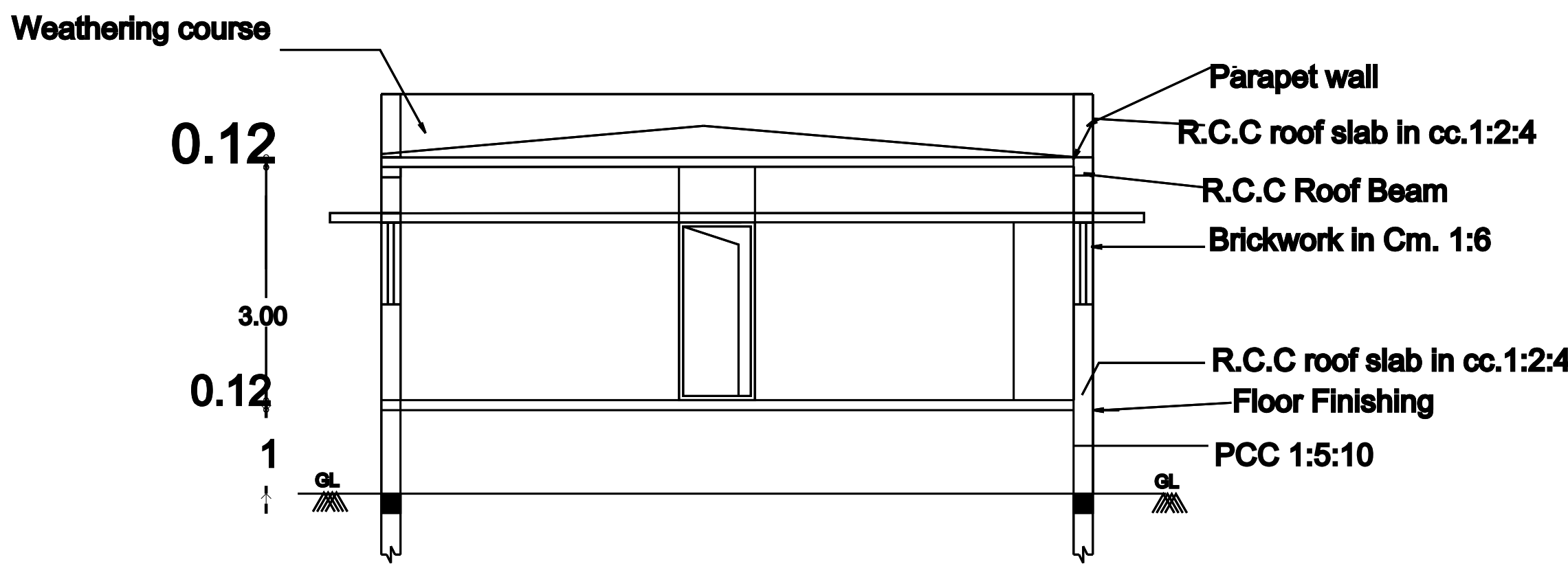
SECTION A-A
