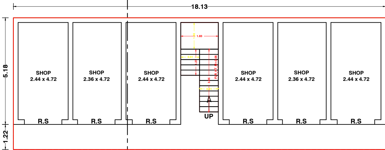
UND FLOOR PLAN
