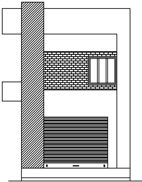
ELEVATION
