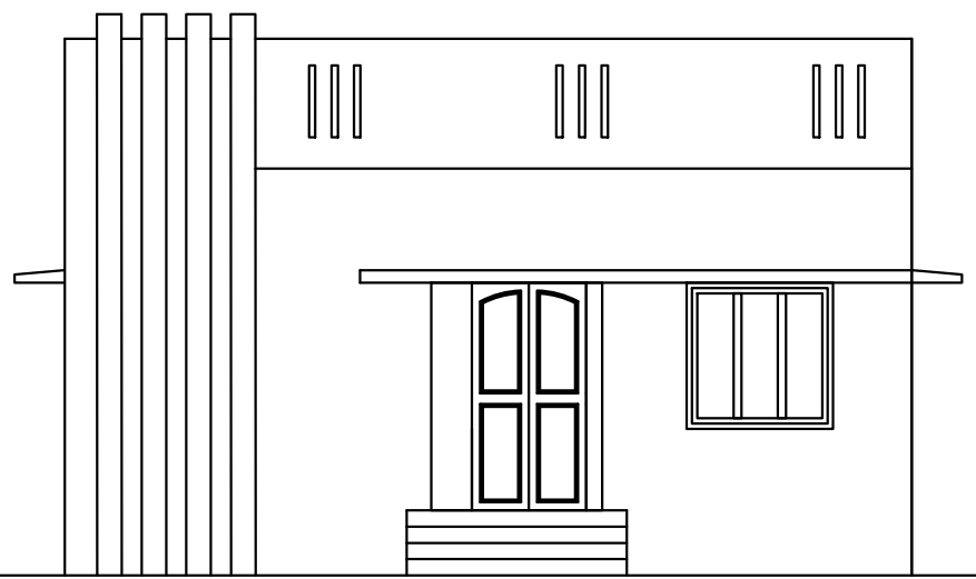
ELEVATION
