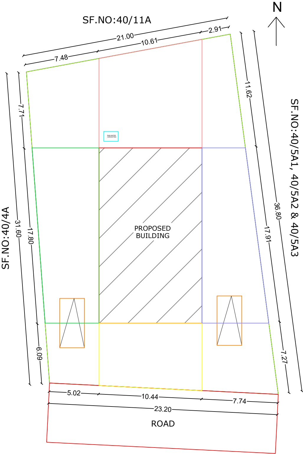
SITE PLAN:1:100
