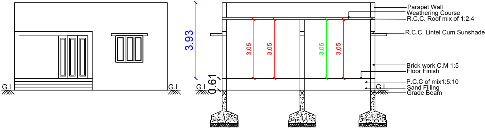
ELEVATION
