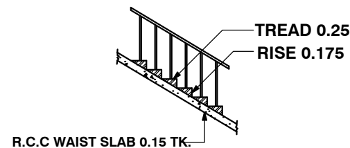
R.C.C WAIST SLAB 0.15 TK.
