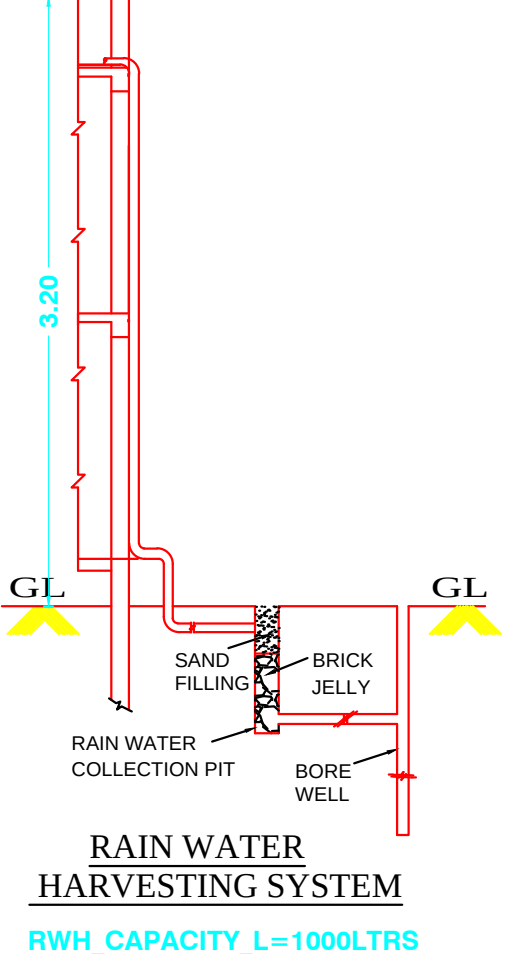
RWH_CAPACITY_L=1000LTRS
