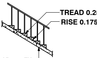
R.C.C WAIST SLAB 0.15 TK
