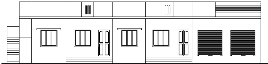
ELEVATION
