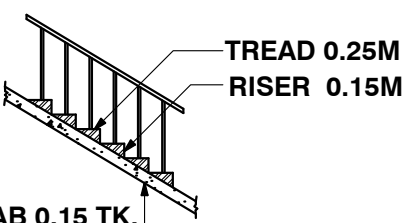
R.C.C WAIST SLAB 0.15 TK.
