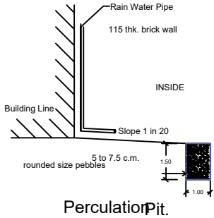
Percolation Pit.
