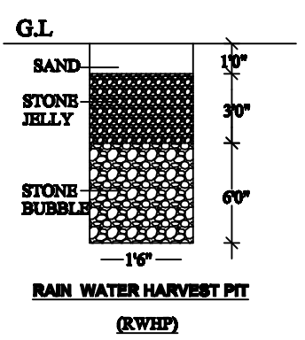
RAIN WATER HARVEST PIT (R.W.H.P)
