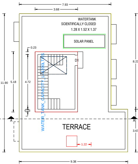
PRO. TERRACE PLAN.
