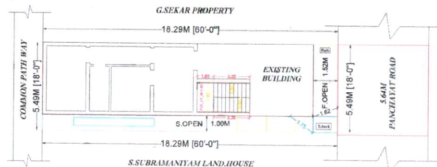
Site Plan. Scale 1:100
