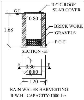
RAIN WATER HARVESTING R.W.H. CAPACITY:1000 Ltr
