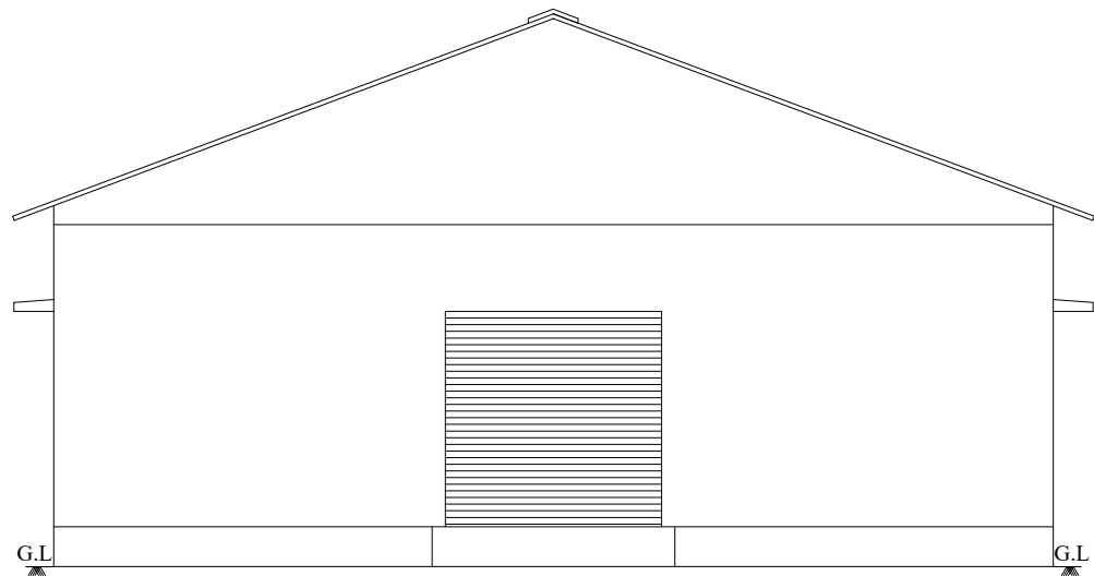
ELEVATION
