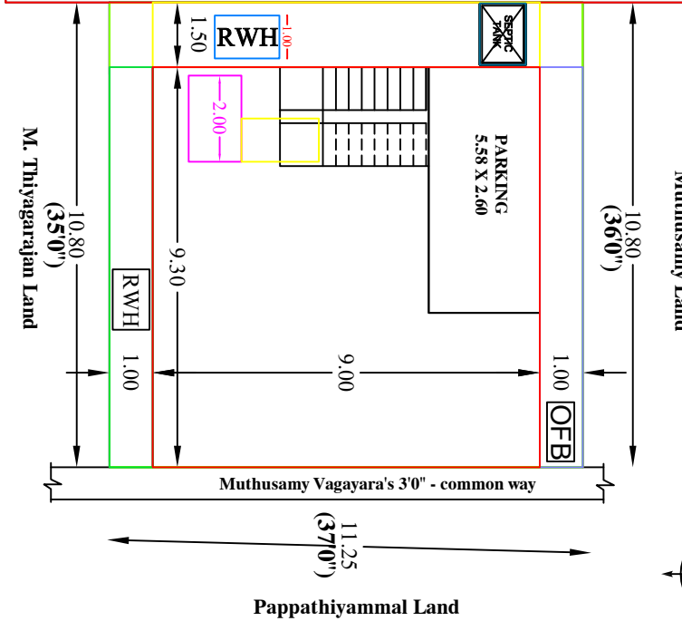
Site Plan.( 1 : 100 )
