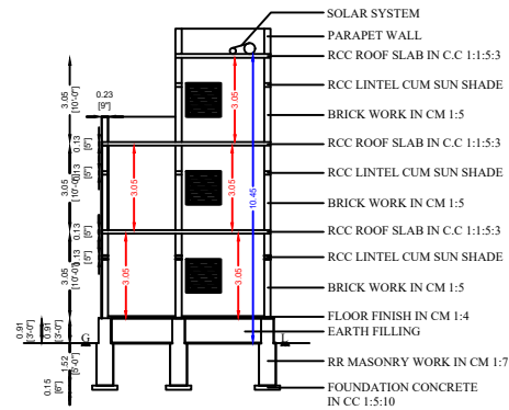
SECTION "AA", "BB" & "CC"
