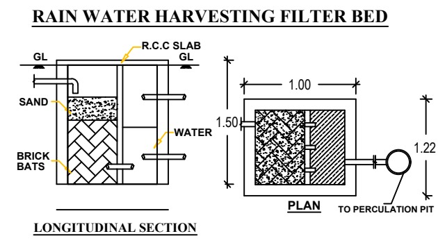
LONGITUDINAL SECTION
