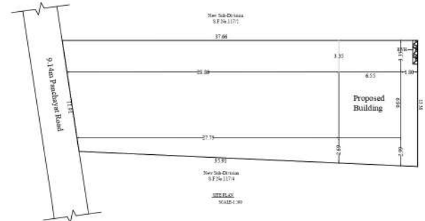
SITE PLAN SCALE - 1:400
