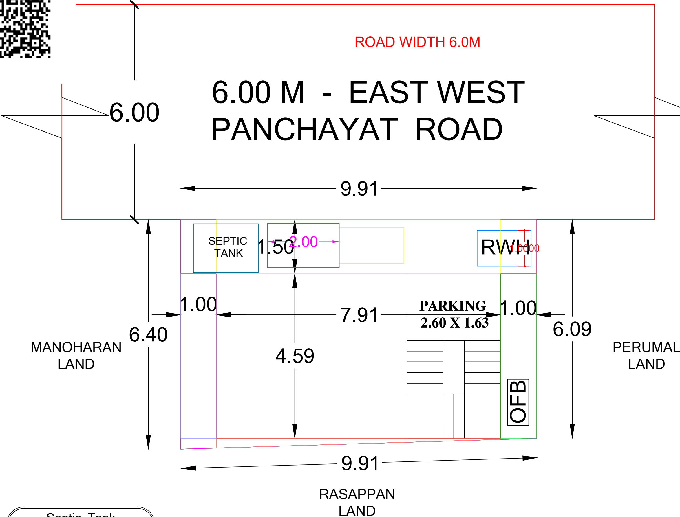
Site Plan.( 1 :100 )
