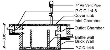
SECTION -SS
