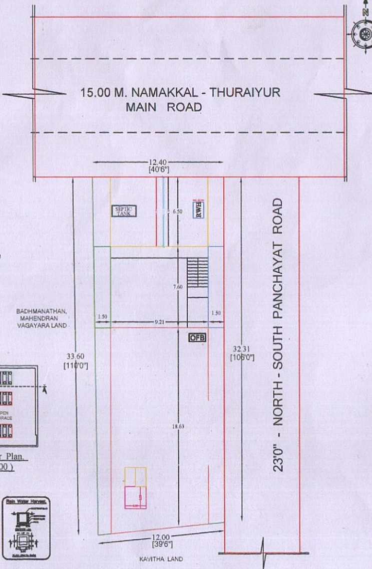
Site Plan. (1:100)
