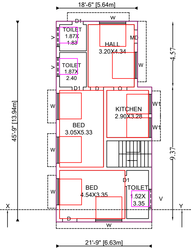
PLAN.
