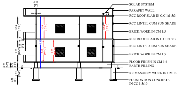
SECTION "AA", "BB"
