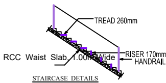
SECTION OHT
