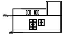
ELEVATION
