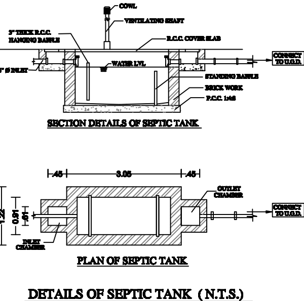
DETAILS OF SEPTIC TANK (N.T.S.)
