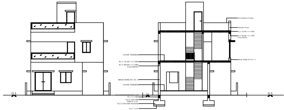
SECTION A-B
