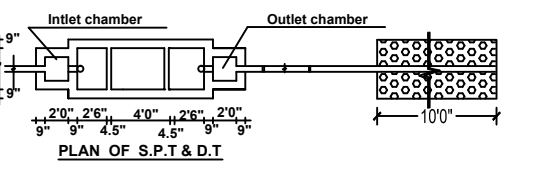
PLAN OF S.P.T & D.T
