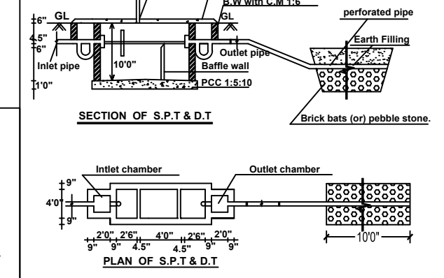
PLAN OF S.P.T & D.T
