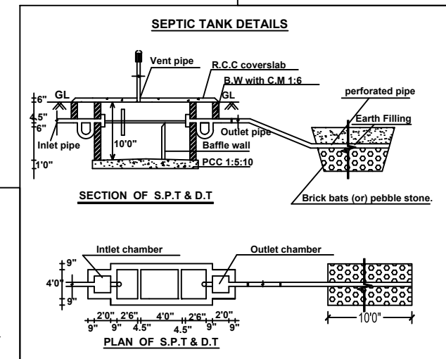
PLAN OF S.P.T & D.T
