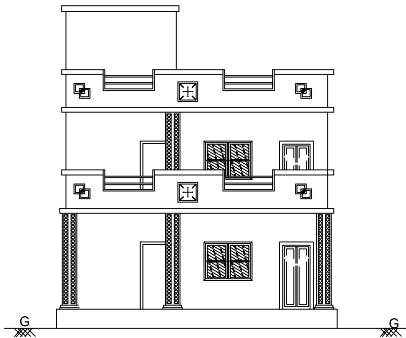
ELEVATION
