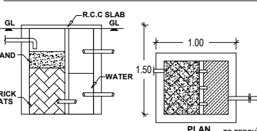
LONGITUDINAL SECTION
