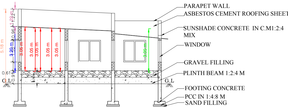
SECTION A-B
