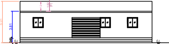
ELEVATION
