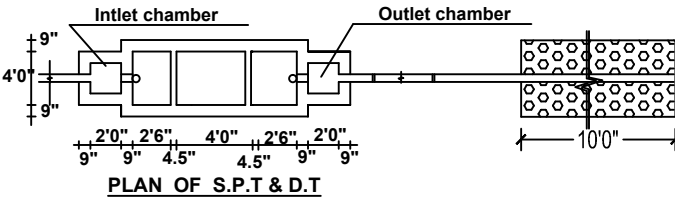
PLAN OF S.P.T & D.T
