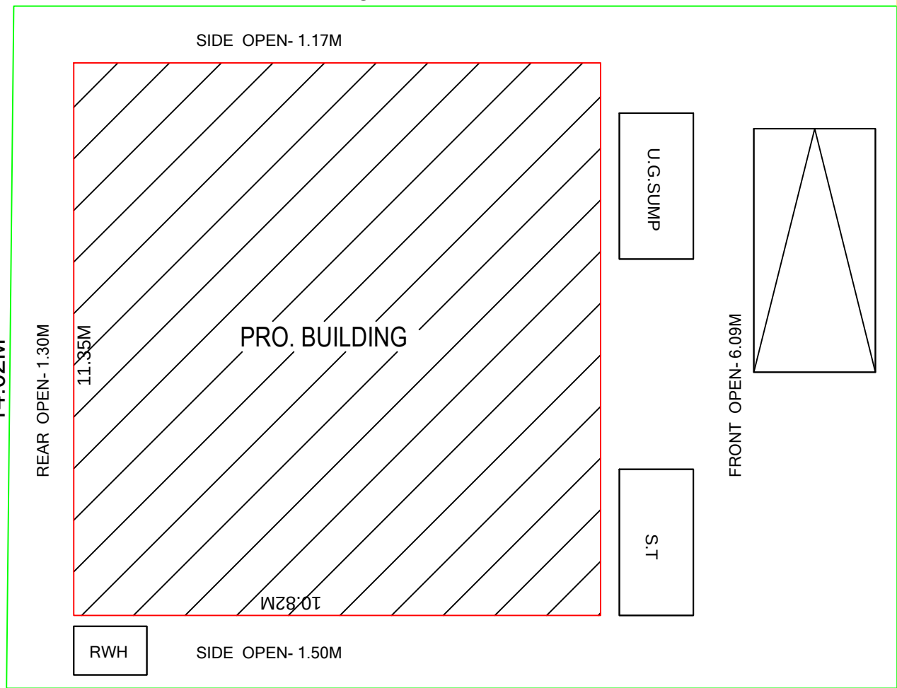
S.F.NO. 142/2 PART AREA SITE PLAN (SCALE -1:100)
