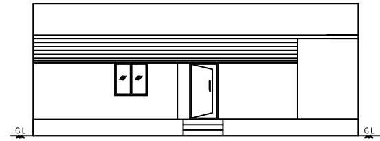
ELEVATION
