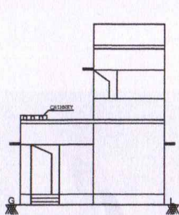
ELEVATION
